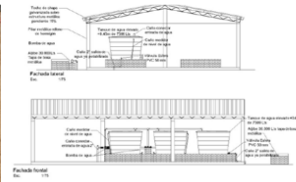
Abastecimiento de agua a la comunidad indígena 2 de Enero, que consistirá en un sistema de bombeo por medio de paneles solares a un tanque elevado; redistribuida a cada domicilio con medidores y administrado mediante un consejo de agua conformado y asistido por la Municipalidad.
